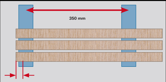
Überstand zu Befestigungspunkt max. 15 mm
