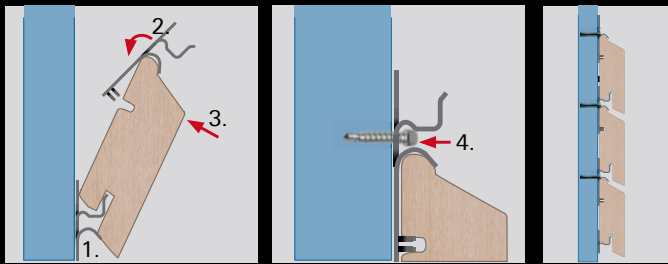
1. Mit dem untersten Profil beginnen. Start Clip an der UK befestigen und Profil einsetzen 2. 2ten Clip am Profil anbringen 3. Profil in Richtung UK eindreihen
