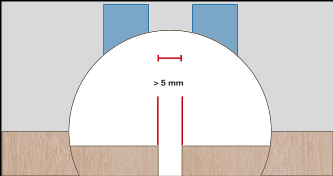
Fuge min. 5 mm
