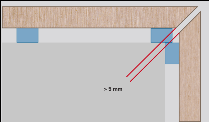
Ecklösung: 90° Gehrung mit Abstand min. 5 mm.
