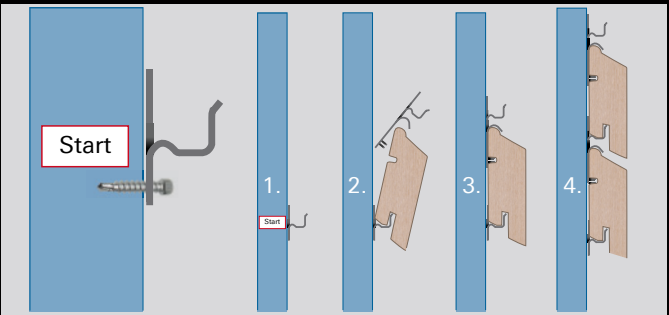
1. Mit dem untersten Profil beginnen. Start Clip an der UK befestigen und Profil einsetzen 2. 2ten Clip am Profil anbringen 3. Profil in Richtung UK eindreihen
