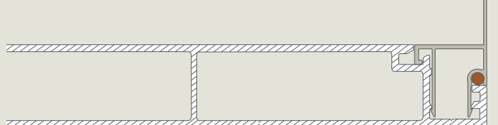
Endprofil mit Aufkantung
