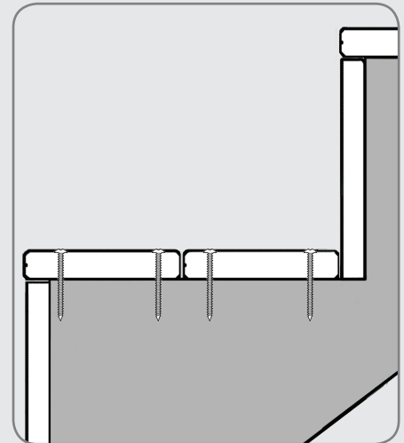
Grundmontage von Treppen
