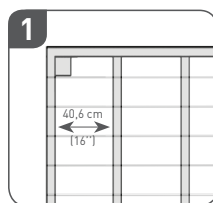
40,6 cm (16") BASISMONTAGE UNTERBAU Maximaler Mittenabstand der Stützbalken 40,6 cm (16"). (30,5 cm (12") Mittenabstand für gewerbliche Anwendungen)
