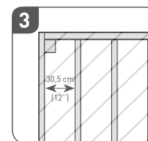
DIAGONALE MONTAGE UNTERBAU Maximaler Mittenabstand der Stützbalken 30,5 cm (12"). Größere Winkel erfordern ggf. kleinere Abstände zwischen den Stützbalken.
