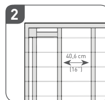
BILDERRAHMEN-UNTERBAU Maximaler Mittenabstand der Stützbalken 40,6 cm (16") plus zusätzliche Stützung des Rahmenzauns (30,5 cm (12") für gewerbliche Anwendungen)
