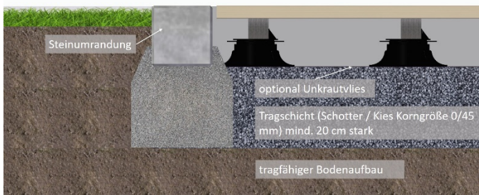
Bild 1. Die Tragschicht sollte ca. 20 cm stark sein.
