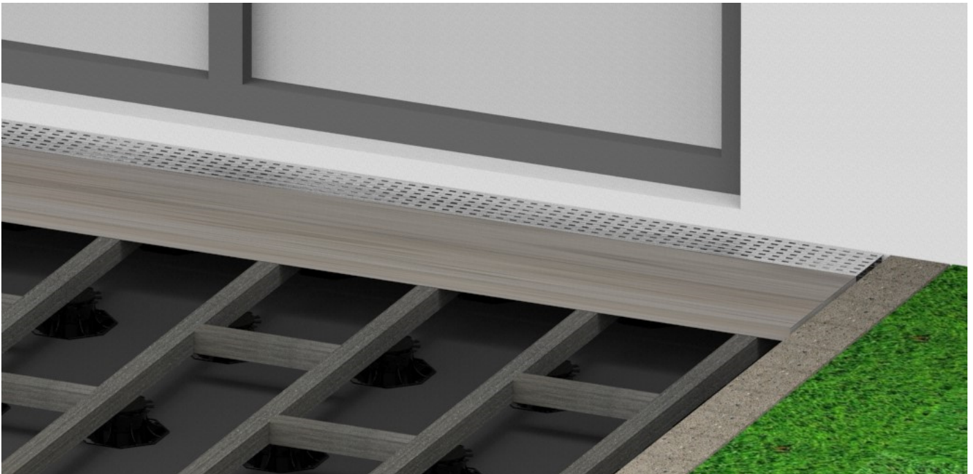
Bild 16. Entwässerungsroste bzw. Rinnen müssen bei geringeren Austrittshöhen < 150 mm eingebaut werden.
