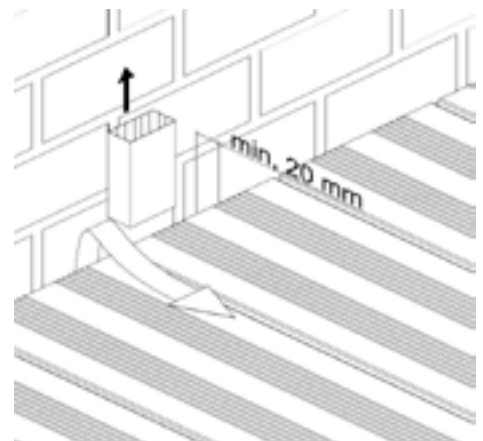
Abb. 2.2 Abstand Randlüftung
