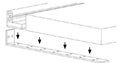
Abb. 2.3 Montage mit Winkelauflege
