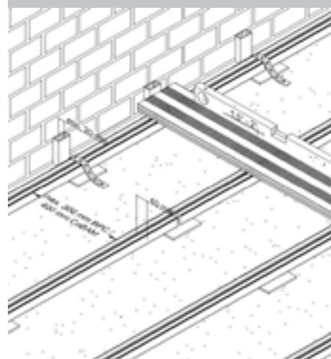
Abb. 3.2 Montage mit geringer Aufbauhöhe
