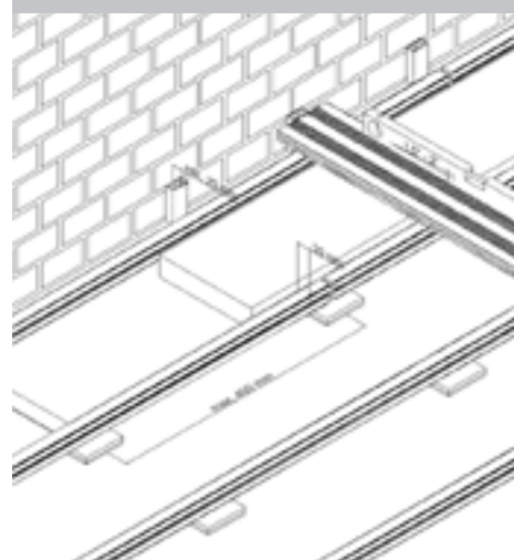
Abb. 3.3 Montage auf Betonplatten
